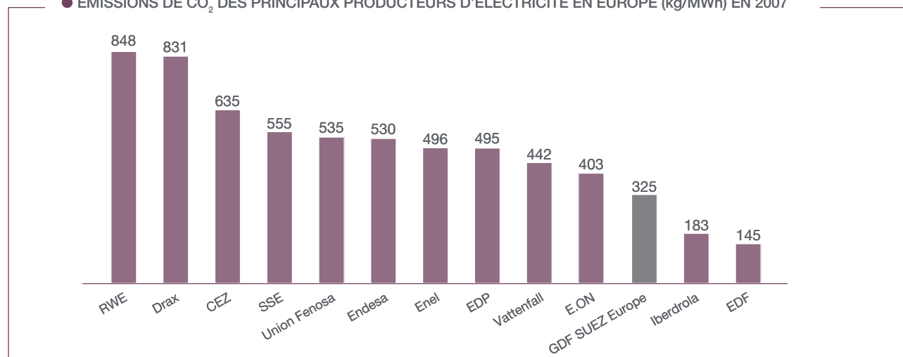
● EMISSIONS DE CO 2 DES PRINCIPAUX PRODUCTEURS D'ÉLECTRICITÉ EN EUROPE (kg/MWh) EN 2007
